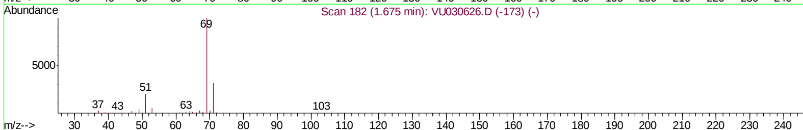
TIC: VU030630.D
